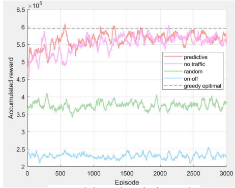
Fig 2. 에피소드별 누적 평균 보상
