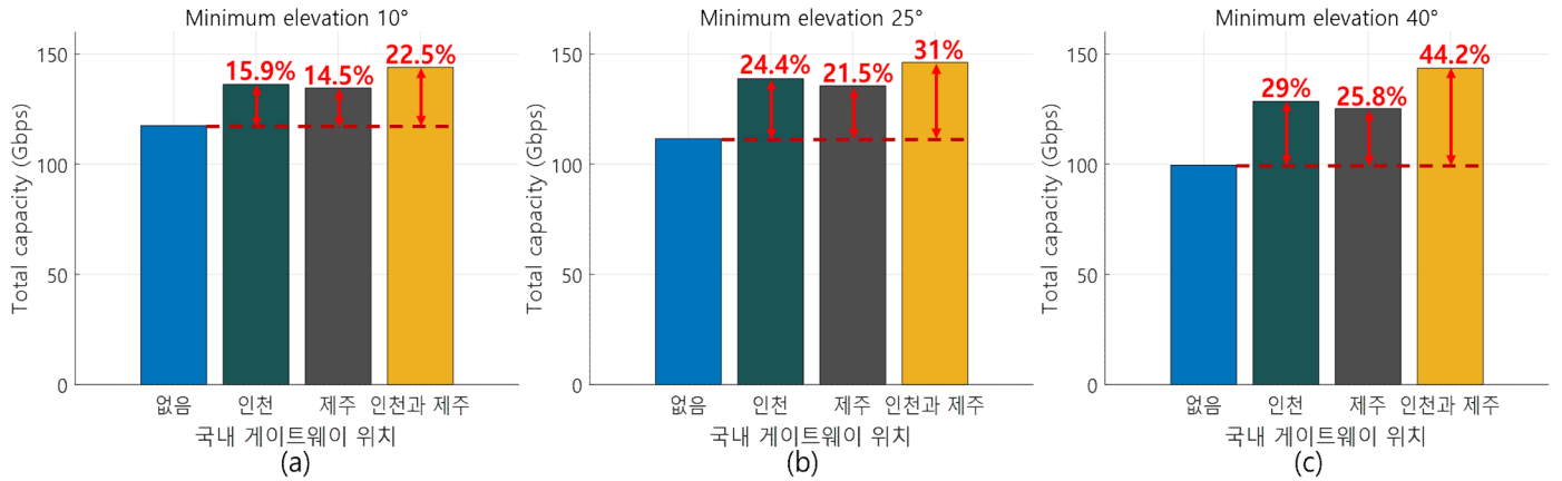
그림 2. 국내 게이트웨이 설치에 따른 총 용량 결과. (a) 최소 고도각이 10°인 경우, (b) 최소 고도각이 25°인 경우, (c) 최소 고도각이 40°인 경우.
