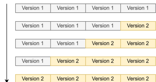
그림 1 롤링 배포
