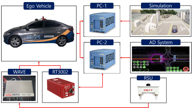
그림 1. Vehicle In the Loop 시스템 구성
