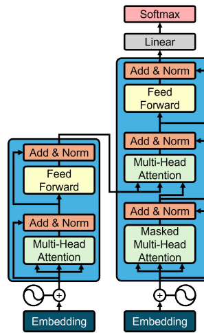
그림 1. Transformer 구조
