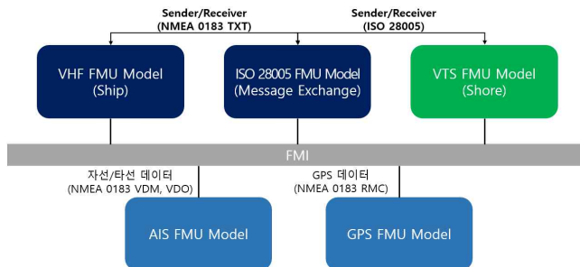
[그림 1] 선박-육상 간 ISO 28005 기반 메시지 교환 구성도(예시)
