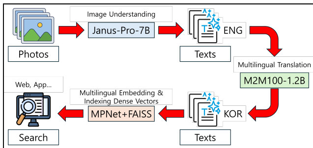
(그림 1) 제안하는 이미지 검색 파이프라인의 전체 구조
