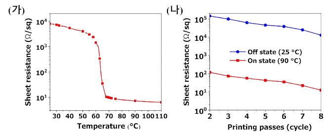
그림 1. (가) 스크린 프린팅된 \text{VO}_2 패턴의 온도별 면저항 측정 결과, (나) 스크린 프린팅 횟수에 따른 \text{VO}_2 패턴의 면저항 측정 결과
