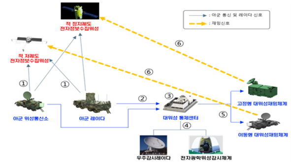
(b) 전자정보수집위성 재밍 운용개념
