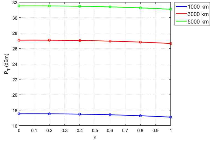
그림 1. 포인팅 오류의 상관계수에 따른 필요 송신 전력
