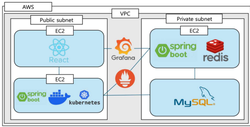
그림 1. 시스템 구조
