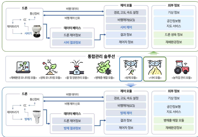
그림 1 밭 작물 재배 정밀 시비 및 방제 모듈 시스템 구성도 Fig 1. Precision fertilization and control module system configuration for field crop cultivation
