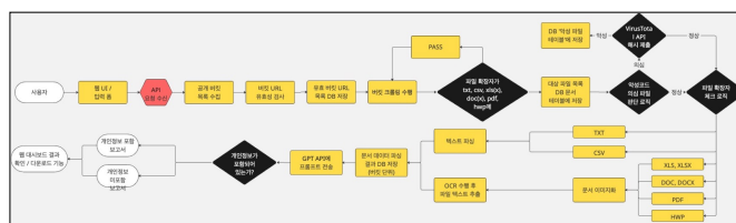
<그림 1> 시스템 플로우차트
