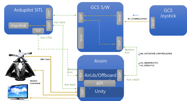
그림 7 공격 영향 실험 구성
