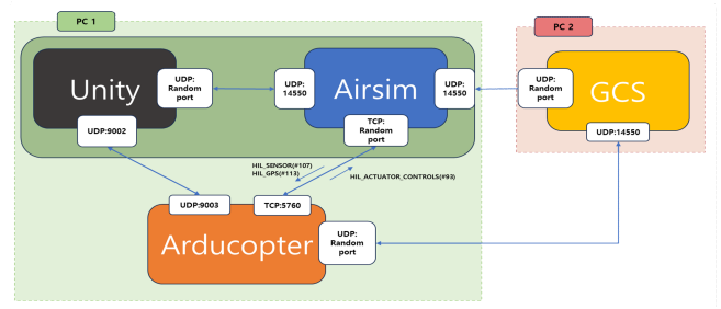
그림 1 SITL 연결 구조
