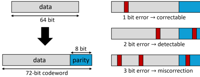
(a) SECCDED 부호어 구성 (b) 비트 오류에 따른 ECC 결과 그림 2. SECCDED ECC 동작 구조
