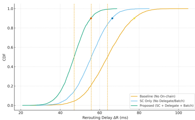
그림 2 재라우팅 지연 \Delta R 의 CDF 비교 결과
