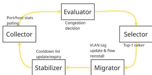
그림 3. 동적 VLAN 재구성 제어 루프
