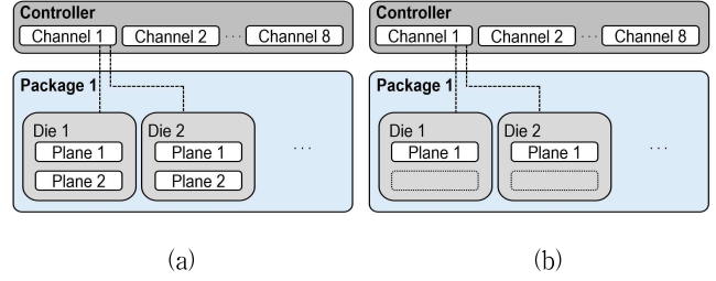
그림 3. NAND 플레인 병렬성 비교. (a) KIOXIA XG6: 채널 - 다이 - 복수 플레인 구조로 플레인 병렬화 가능 (b) NVMeVirt: 다이당 플레인=1로 단 순화되어 내부 병렬성 부재.
