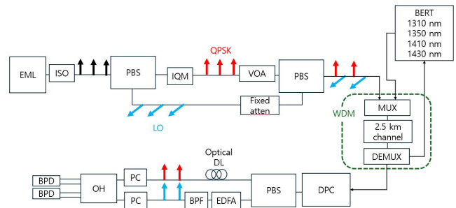
Figure 1: CV QKD 구현 다이어그램
