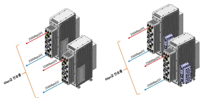
그림 1. Gbps급 데이터링크 단말 구성 (좌 : 출력증폭반 탈착 형상, 우 : 출력증폭반 장착 형상)
