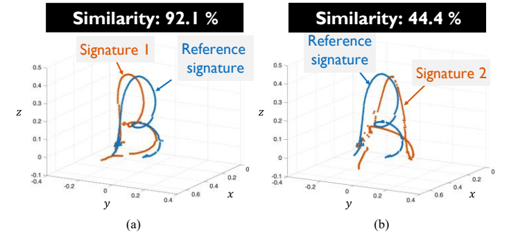
그림 4. 유사도 판별 결과. (a): 레퍼런스와 동일한 서명이 입력된 경우, (b): 레퍼런스와 상이한 서명이 입력된 경우.
