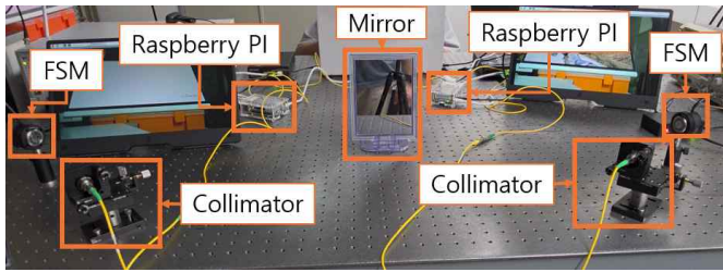
그림 2 장애물 회피형 무선 광통신 구현
