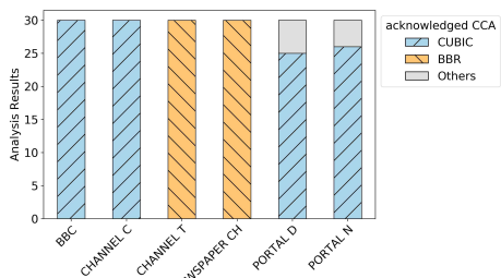
<그림 8> Delay 200ms에서의 CCA 분석 결과
