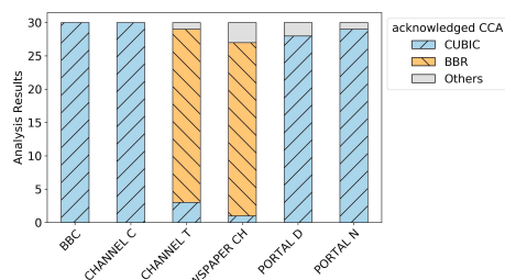
<그림 6> Delay 100ms에서의 CCA 분석 결과
