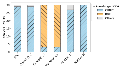
<그림 7> Delay 150ms에서의 CCA 분석 결과
