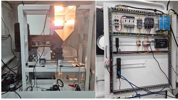
그림 2. RVM 초분광 분류 시스템
