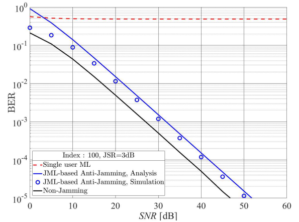
그림 1 SLJ 공격 환경에서 JML 검파 기반 항제밍 기법의 BER 성능
