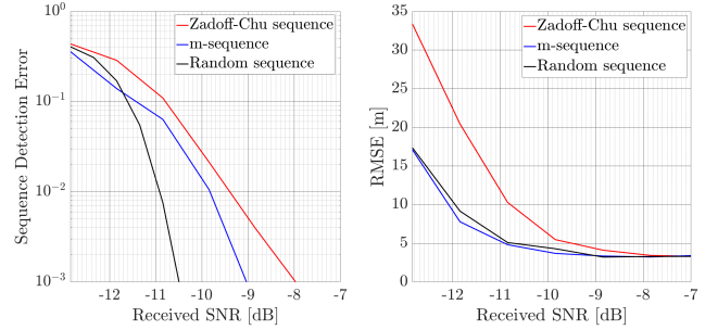
그림 2. OFDM-ISAC 시스템의 통신 및 측위 성능
