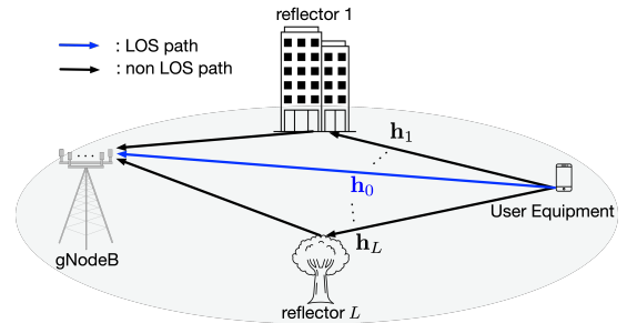
그림 1. 5G NR 프리앰블 기반 OFDM-ISAC 시스템 모델
