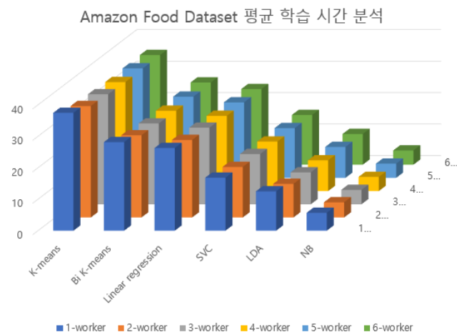
그림 1 Amazon Food Dataset 학습 시간 분석
