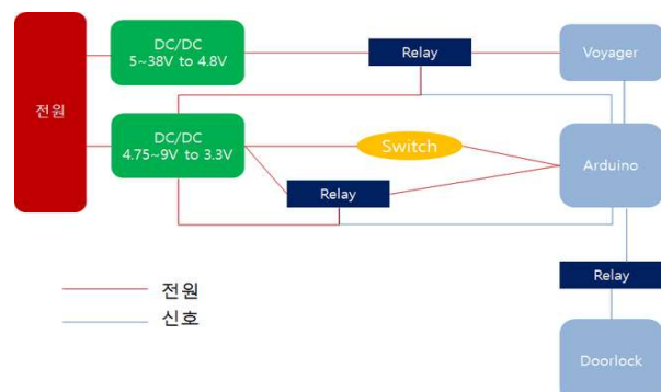
그림 1. 설계 개념도
