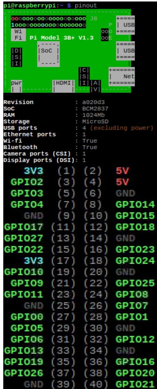
[그림1] pinout을 통해 확인할 수 있는 Raspberry Pi의 정보
