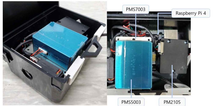
그림 4. 구현된 미세먼지 측정 모듈
