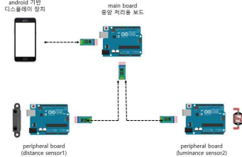
그림 3 시험 시나리오의 시스템 구성도
