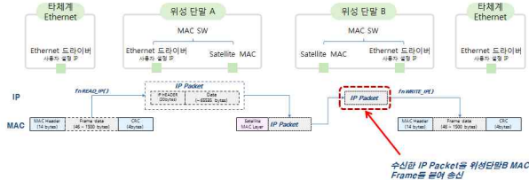
그림 7. 다중망 구조에서의 IP 패킷처리 흐름
