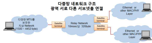
그림 5. 레이어3로 운용시 네트워크 구조
