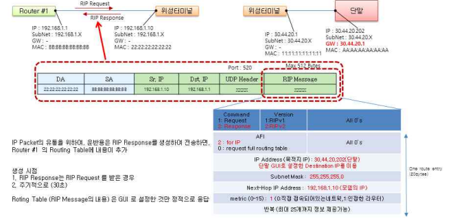
그림 9 RIP(Routing Information Packet) v2 의 Response Packet구현
