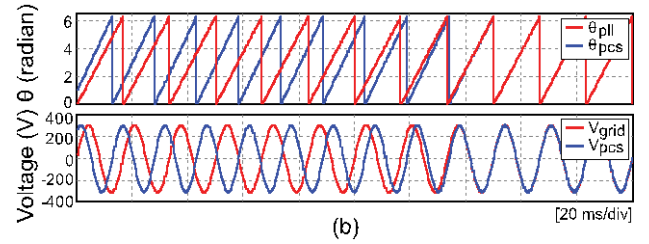
그림 4. 슬루율 조절이 가능한 위상 동기화기: (a) 구성 (b) 시뮬레이션
