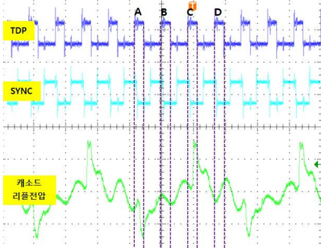
그림2. 신호 비동기화 시 캐소드 리플전압
